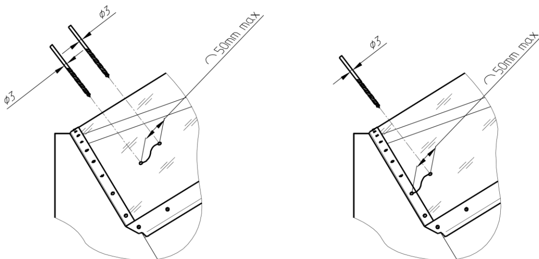
Fig. 10 : perçage des vitres pour stopper les criques
